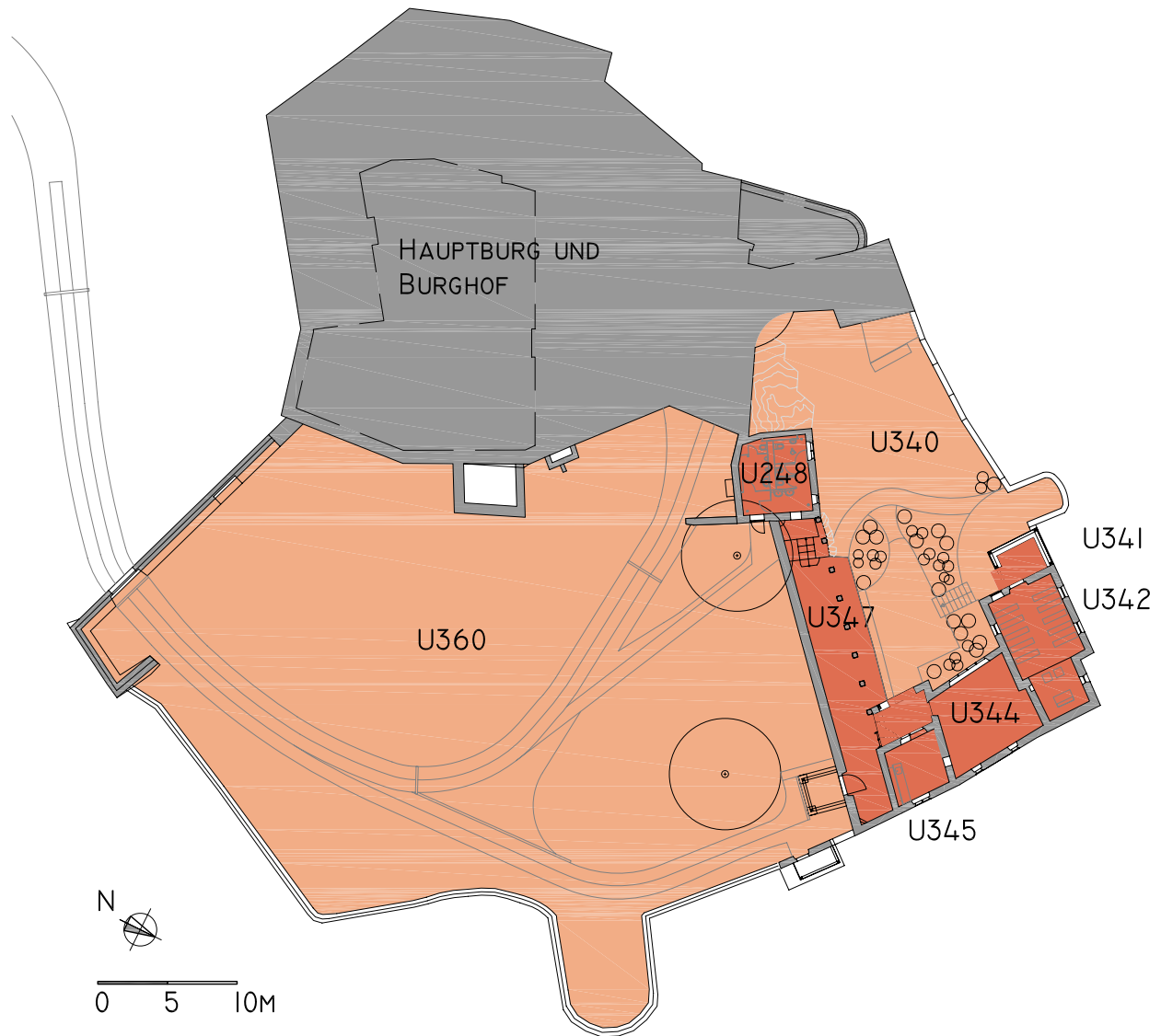
GRUNDRISS ROSENGARTEN UND KAPELLENBAUTEN EBENE U3 - U2 M 1:500
